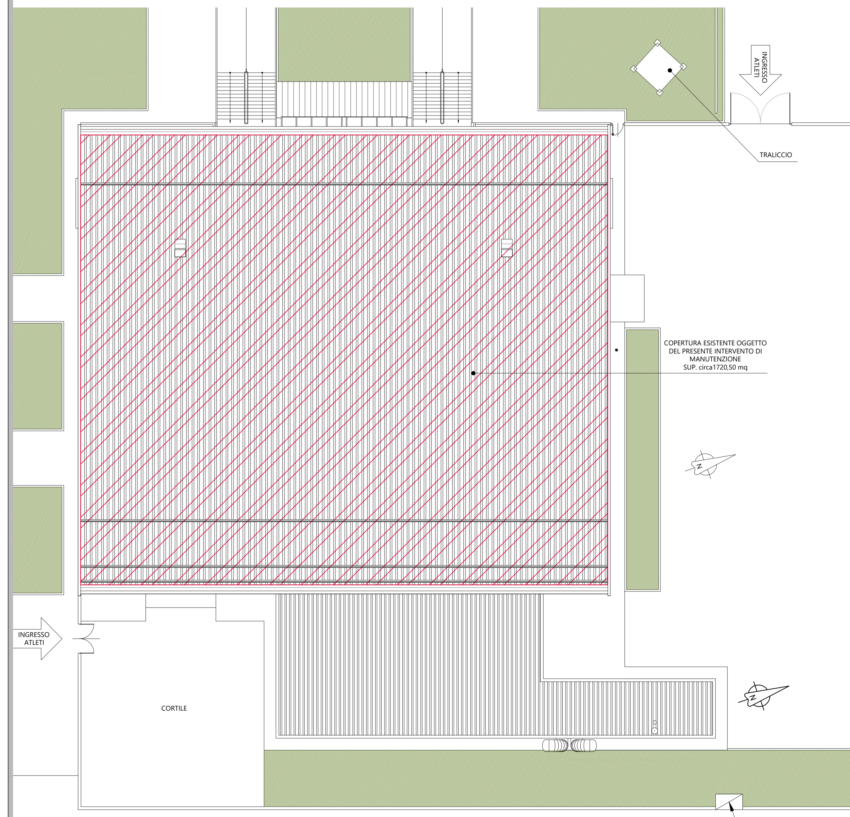
PLANIMETRIA COPERTURA scala 1:200
