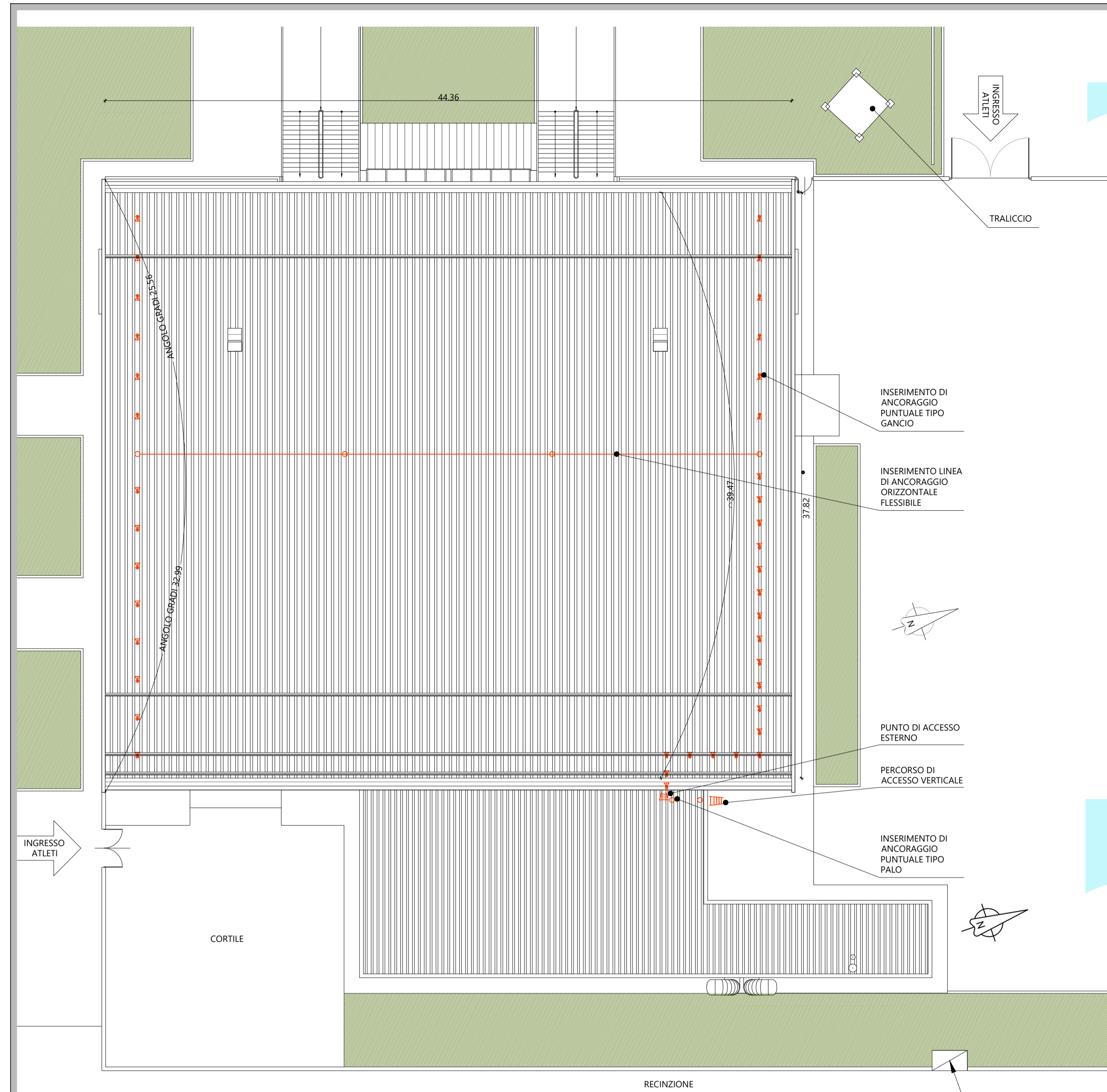
PLANIMETRIA COPERTURA con individuazione punti di ancoraggio per manutenzione scala 1:200
